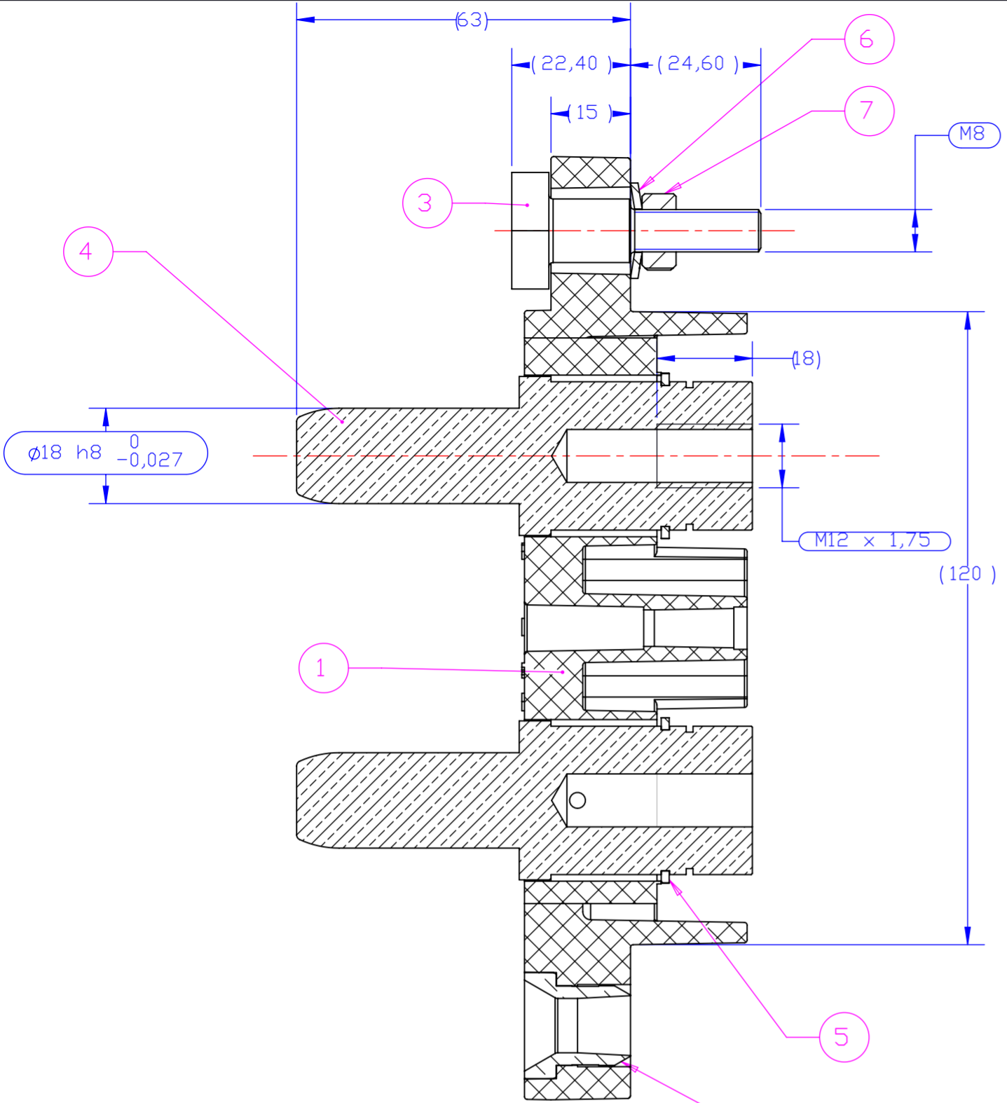
COUPE E-E
